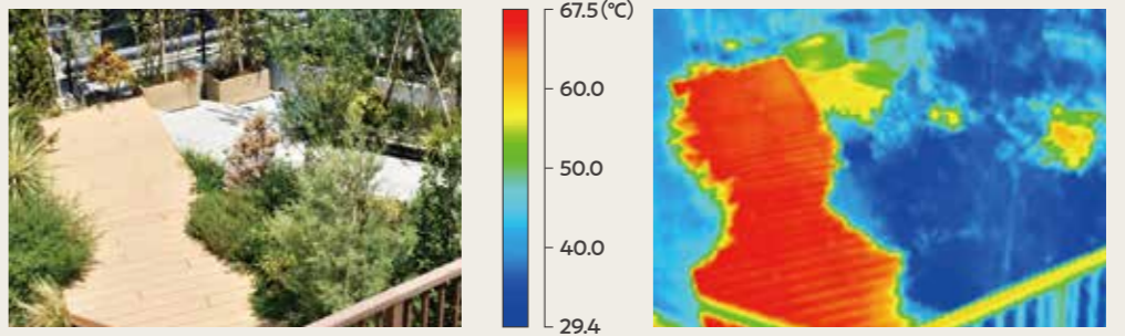
田島ルーフィング 小台研修センター 屋上緑化 10ページ掲載の屋上緑化展示場を、赤外線サーモグラフィで計測してみました。 緑化面積 164.21m 2 計測日 2023年7月26日 上:ハーブエリア付近 下:多目的広場付近
